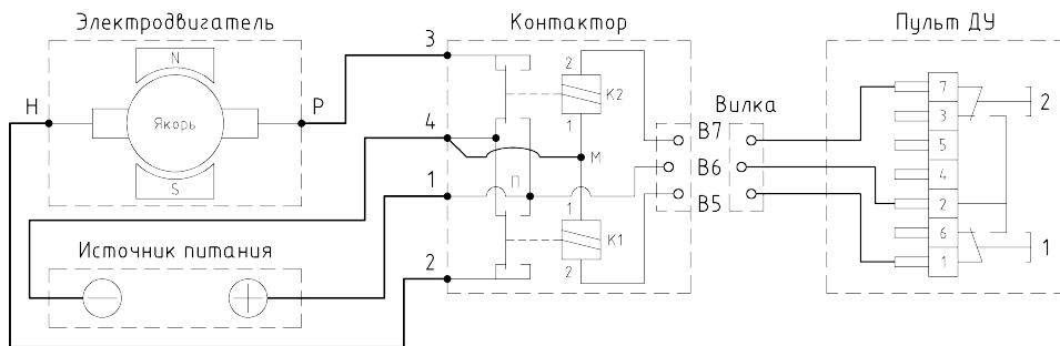
Рис. 2. Принципиальная электрическая схема при управлении электродвигателем с постоянными магнитами.
